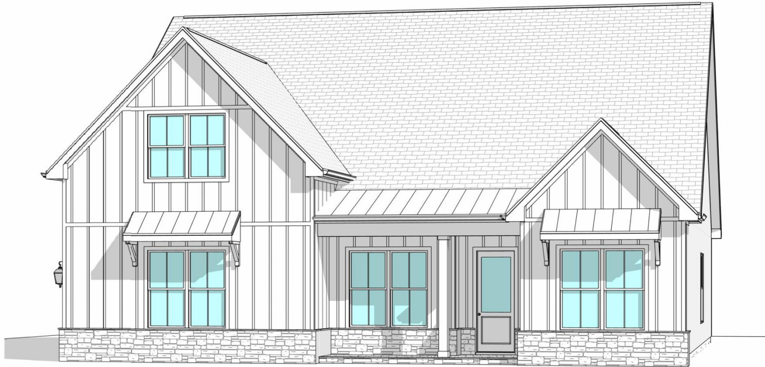
Elevation B
