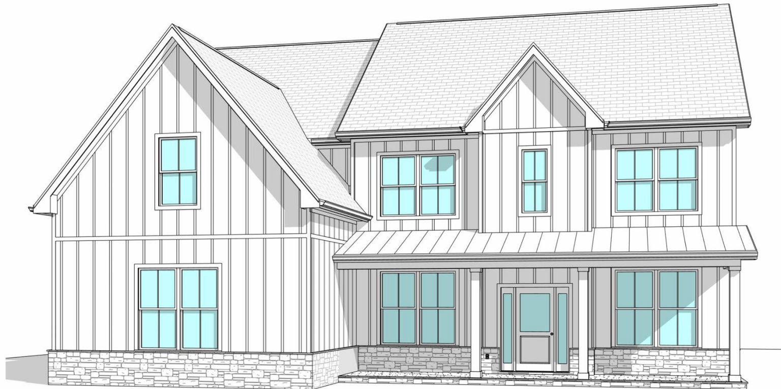
Elevation B
